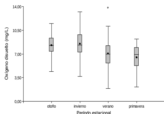
Fig. 4: Gráfico Box plot. Variación temporal del oxígeno disuelto.
