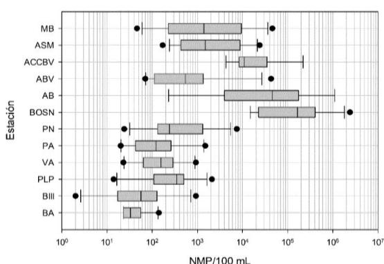
Fig. 7: Gráficos box-plot de E. coli (periodo 2008-2012).
