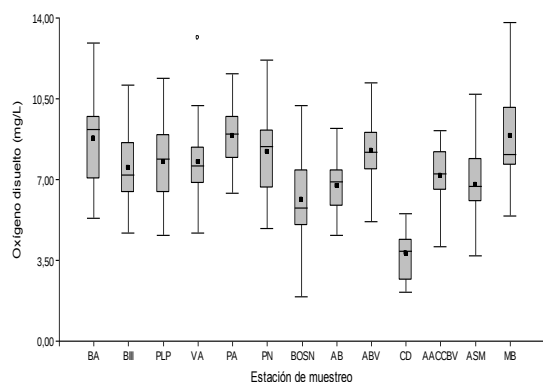
Fig. 3: Gráfico Box plot. Variación espacial del oxígeno disuelto.
