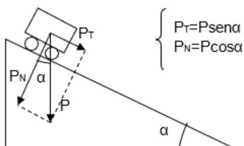
Figura 3.9: La fuerza que acelera en un plano inclinado es la componente tangencial (paralela al plano inclinado) del peso.
