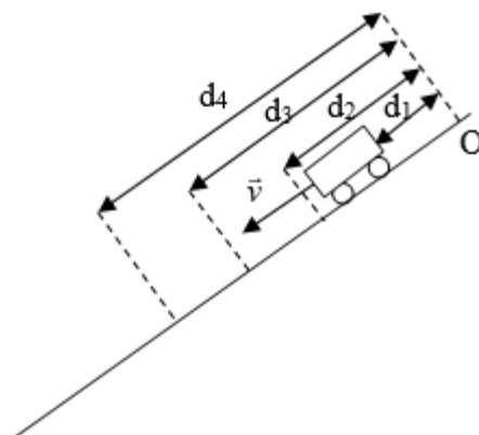
Figura 2.8: El experimento que realizó Galileo para estudiar la relación entre el espacio que recorría un cuerpo y el tiempo que tardaba en recorrerlo, en un plano inclinado.
