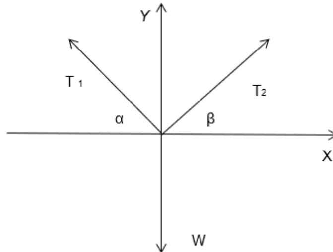
Figura 1.19: Diagrama de cuerpo libre
