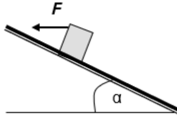
Figura 3.29: Representación del problema 11.
