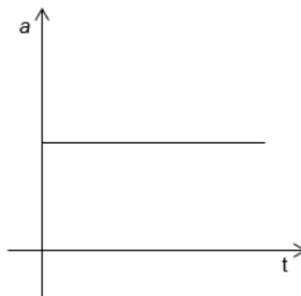
Figura 2.23: Función aceleración: una constante en el MRUV.
