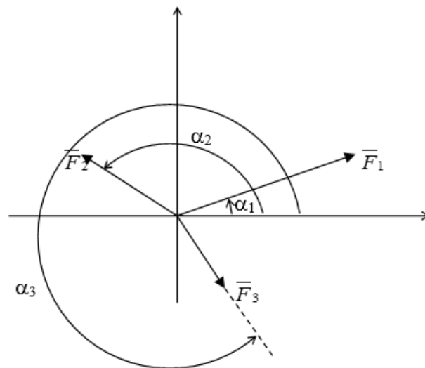
Figura 1.12: Ubicación de los vectores en un sistema de ejes
