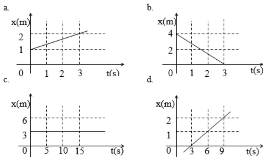
Figura 2.19: Distintos casos de movimiento rectilíneo uniforme.
