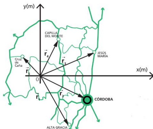
Figura 2.6: Vectores posición que precisan sobre el lugar que ocupan determinadas ciudades o accidentes geográficos en relación a una localidad de referencia.
