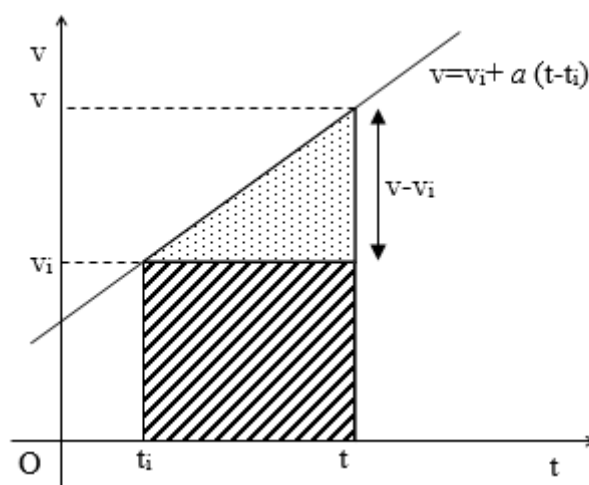
Figura 2.21. El área rayada indica el espacio recorrido entre los instantes de tiempo t_i y t . Calculando el área para valores genéricos se encuentra la función posición.
