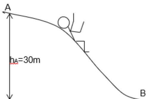
Figura 3.26: Representación del problema 8.
