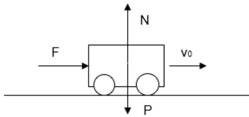
Figura 3.4: La fuerza aplicada sobre el cuerpo, posee la misma dirección que la velocidad que lo anima.
