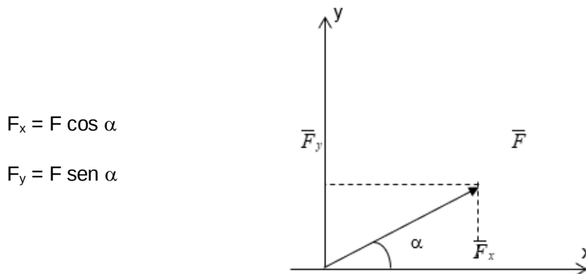
Figura 1.11: Proyección de un vector sobre los ejes.
