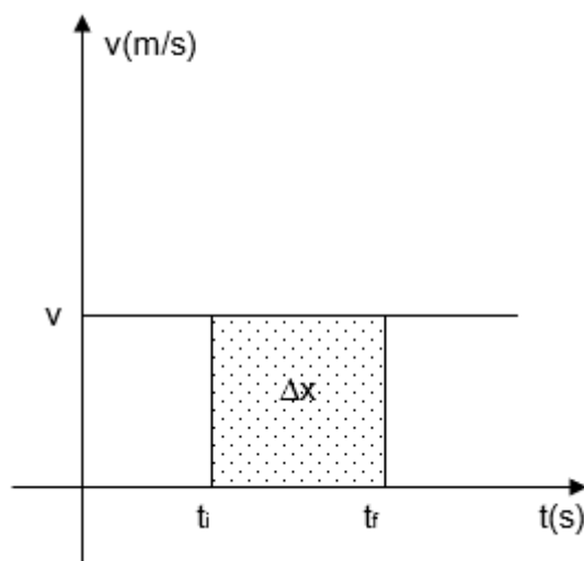
Figura 2.18: Función velocidad y significado físico del área encerrada entre la función velocidad y el eje de los t .
