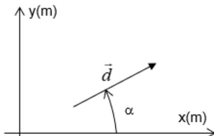
Figura 1.6: Vector representado en un sistema de ejes cartesianos
