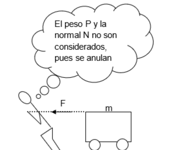
Figura 3.19: Representación del problema 1.
