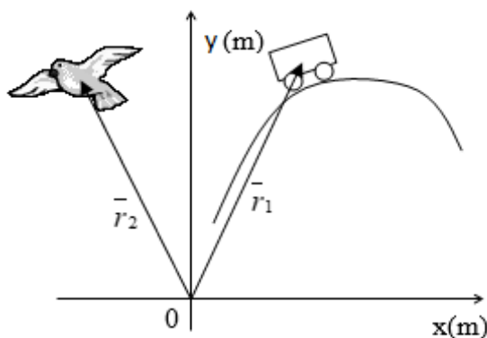
Figura 2.5: Vectores posición.
