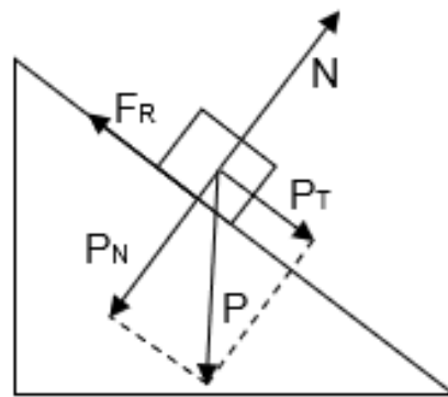
Figura 3.10. La fuerza normal es siempre perpendicular al plano tangente a la superficie en el punto considerado y se anula con la componente normal de la fuerza aplicada
