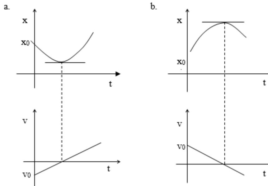
Figura 2.22. Cada caso muestra las funciones posición y velocidad de un cuerpo.
