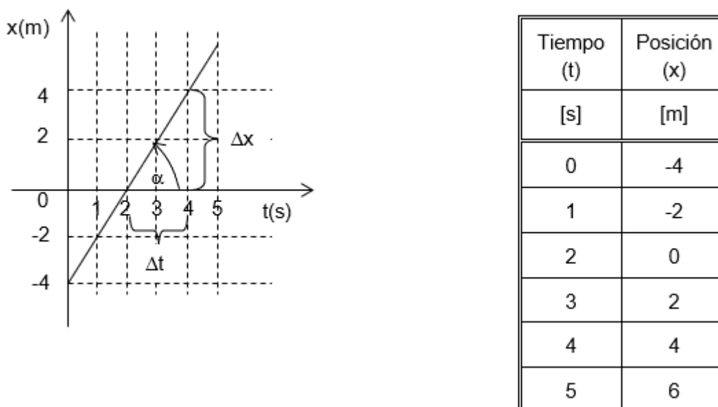
Figura 2.17. Representación gráfica de la función posición y tabla correspondiente a un MRU.
