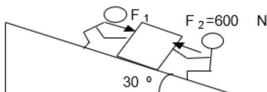
Figura 3.34: Representación del problema VIII.
