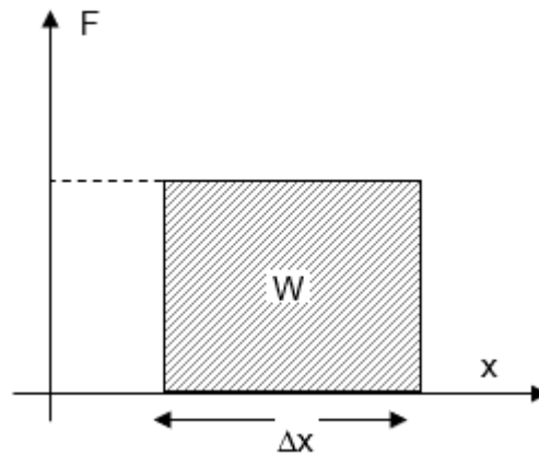
Figura 3.13: Representación gráfica del trabajo mecánico.
