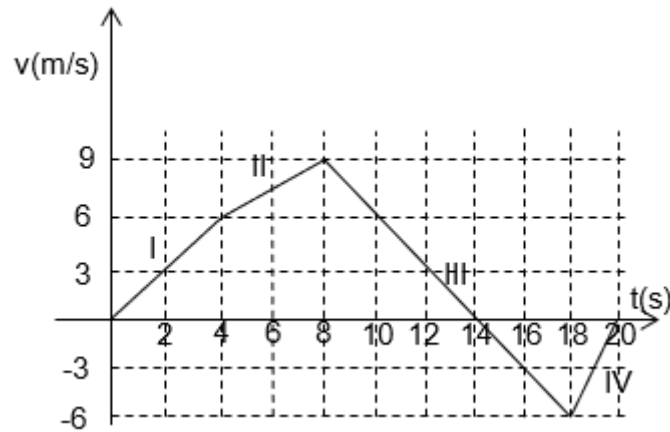
Figura 3.20: Representación del problema 2.
