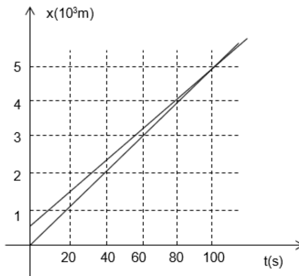
Figura 2.25: Forma gráfica de resolver un sistema de ecuaciones.
