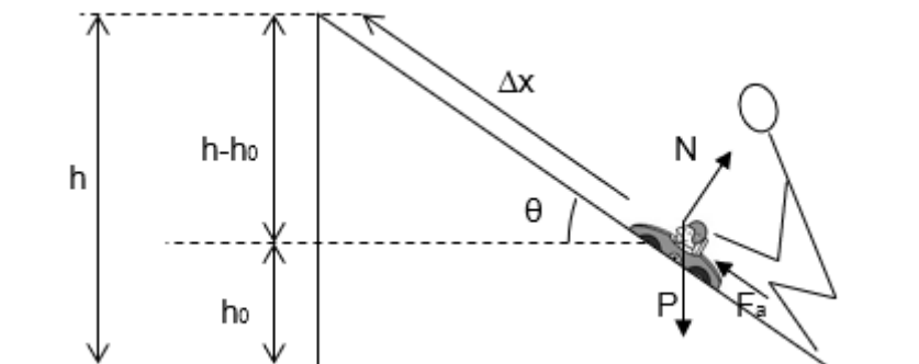
Figura 3.17: El cochecito de juguete está sometido a su peso, una fuerza normal y una fuerza aplicada \vec{F}_a . Por definición, \sin \Delta = (h - h_0) / \Delta x , de modo que \Delta x \cdot \sin \theta = (h - h_0) .
