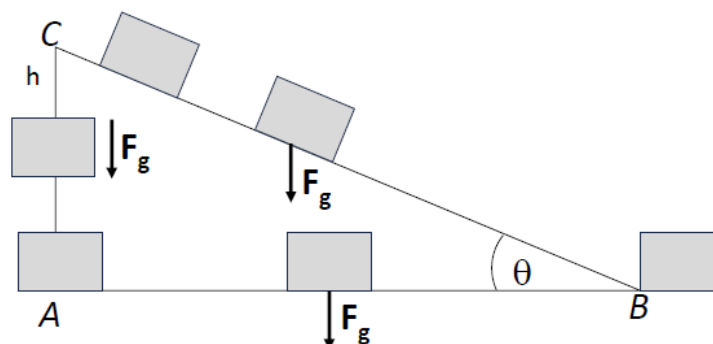
Figura 3.18: El cochecito de juguete está sometido a su peso, una fuerza normal y una fuerza aplicada \vec{F}_a . Por definición, \sin \Delta = (h - h_0) / \Delta x , de modo que \Delta x \cdot \sin \theta = (h - h_0) .
