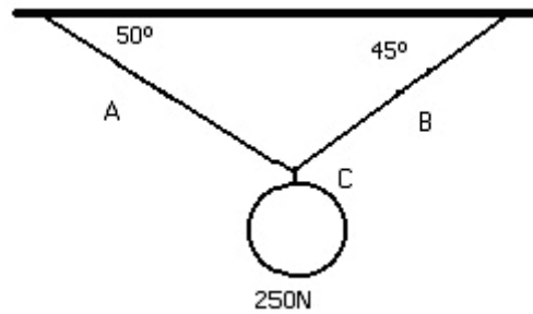
Figura 1.20: Sistema de fuerzas en equilibrio
