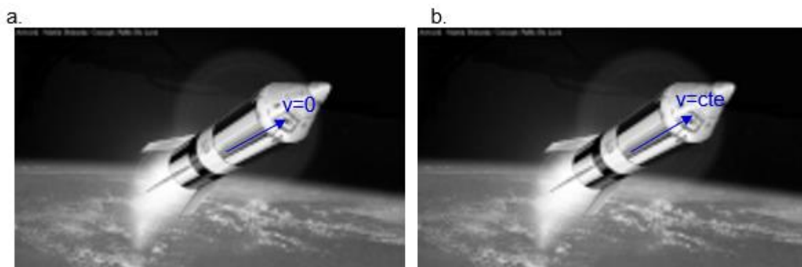
Figura 3.1: Un cuerpo ubicado en una zona del espacio en la cual la gravedad es nula, y por tal motivo no actúan fuerzas sobre el mismo. En a. está en reposo, por lo cual se mantendrá con velocidad nula; en b. como el cuerpo tiene cierta velocidad, la mantiene constante.
