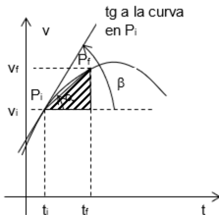
Figura 2.16: Aceleración instantánea
