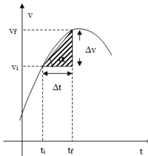
Figura 2.15: Interpretación gráfica de la aceleración media.
