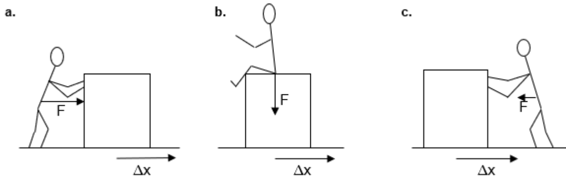
Figura 3.14: Un hombre aplica una fuerza a un mueble con distintas direcciones. En (c) podemos imaginar que el mueble está siendo frenado y llevado al reposo.
