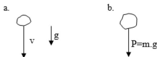
Figura 3.8: Un cuerpo en caída libre experimenta una aceleración, y la dinámica interpreta como que sobre el cuerpo actúa una fuerza. A esta fuerza se la denomina fuerza peso.
