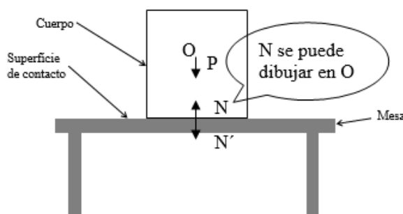
Figura 3.6: Por acción de la gravedad, sobre el cuerpo aparece la fuerza peso; en la superficie de contacto entre el cuerpo y la mesa aparece un par de fuerzas de acción y reacción.
