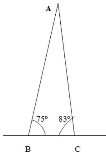
Figura 1.15: Construcción del triángulo
