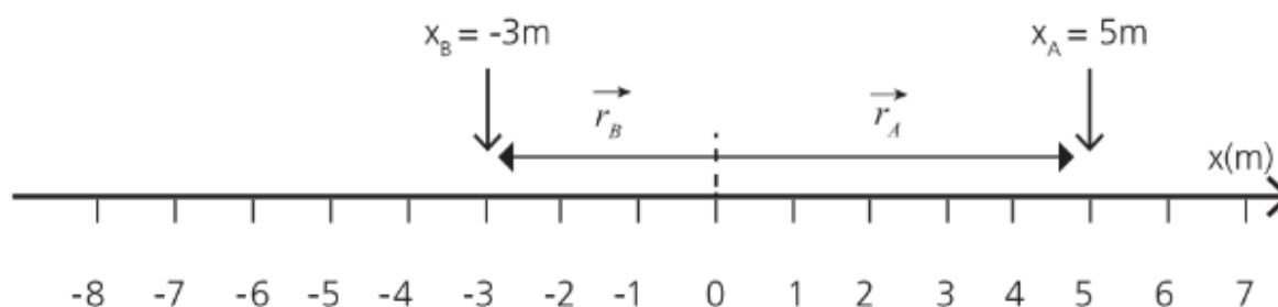
Figura 2.10: Posición de dos partículas (cuerpos A y B) que se mueven según una trayectoria rectilínea.
