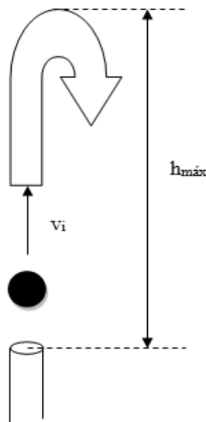
Figura 2.27: Tiro vertical: se advierte una primera parte en la cual el cuerpo sube desacelerado y otra, en la cual el cuerpo baja acelerado
