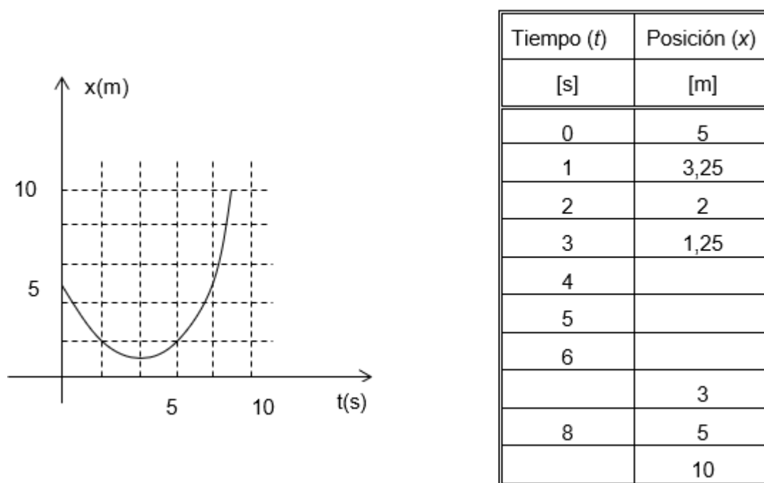
Figura 2.11. Función posición.
