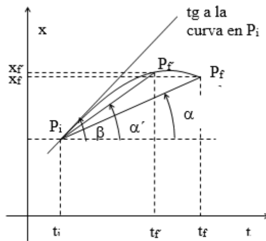
Figura 2.14: Velocidad instantánea.
