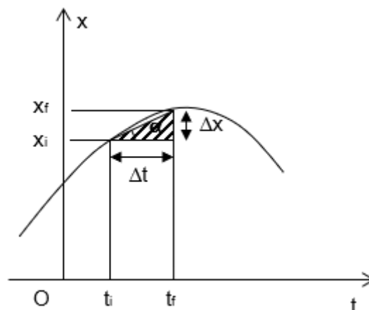
Figura 2. 13. Interpretación gráfica de la velocidad media.
