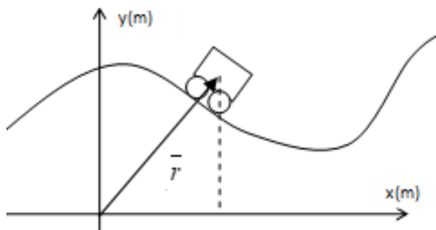
Figura 2.4: Vector posición
