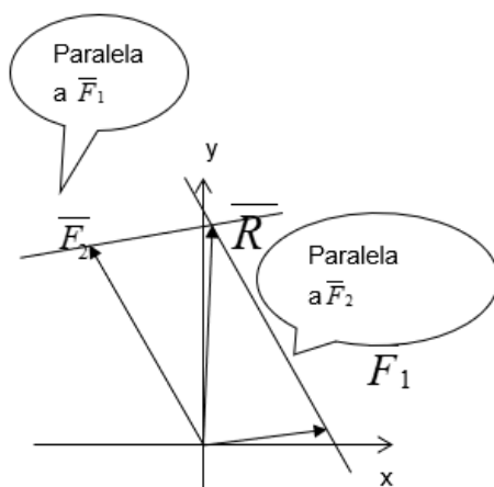
Figura 1.9: Método gráfico para sumar vectores
