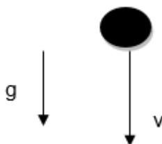
Figura 2.26. Caída libre de un cuerpo
