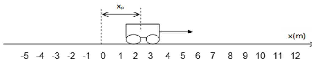
Figura 2.9: Movimiento rectilíneo de un cuerpo y sistema de coordenadas elegido para estudiarlo.
