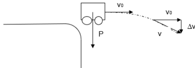
Figura 3.5: La fuerza aplicada sobre el cuerpo no posee la misma dirección que la velocidad que lo anima, por lo cual el movimiento en general será curvilíneo.
