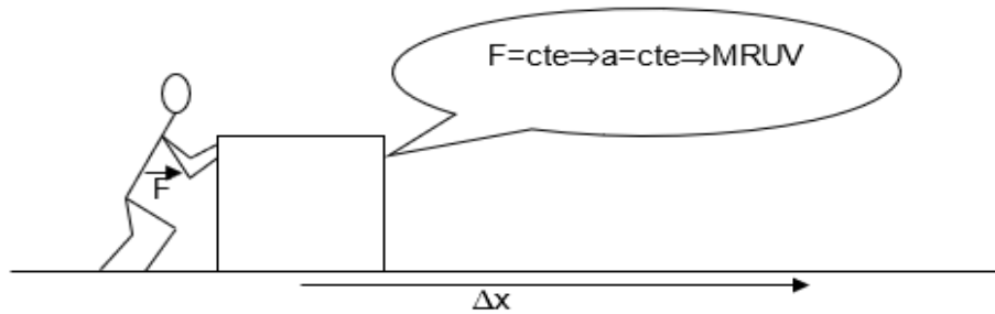
Figura 3.16: Una fuerza \vec{F} realiza trabajo sobre un objeto cuando éste se desplaza una distancia \Delta\vec{x} . La velocidad varía de \vec{v}_i a \vec{v}_f .
