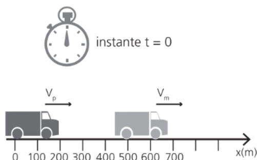
Figura 2.24: Esquema de la situación planteada
