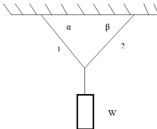
Figura 1.18: Esquema de la suspensión de un cuerpo mediante dos cuerdas
