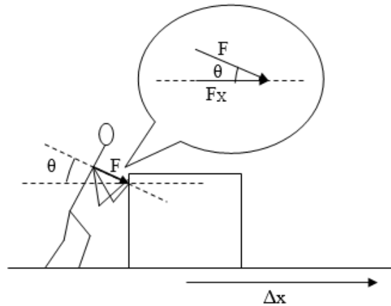
Figura 3.12: Trabajo efectuado por la fuerza \vec{F} que actúa mientras el cuerpo se desplaza \Delta x .
